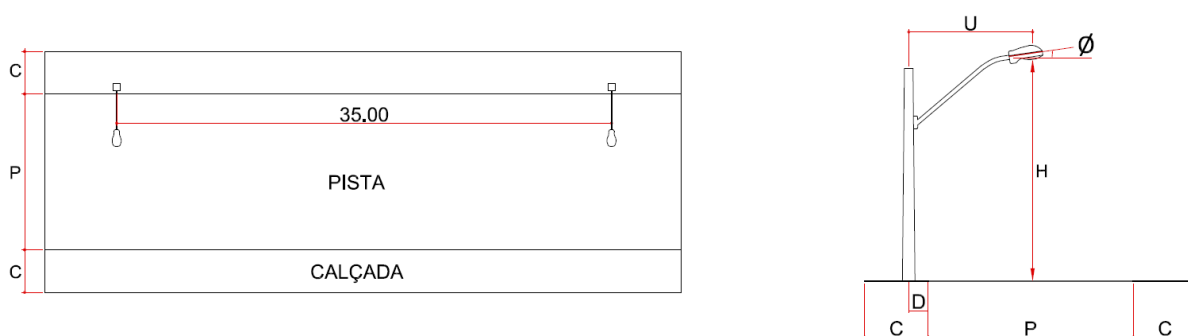
Figura 1 – Cenário genérico de simulação para V3 (sem escala).
